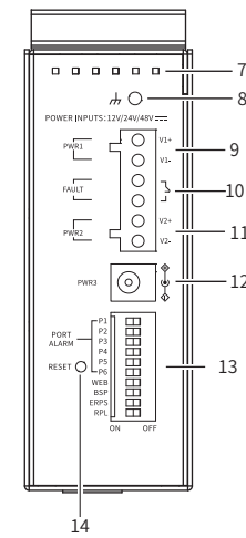
TL-SG2206R工业级 上面板示意图
