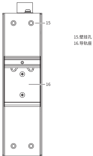
TL-SG2206R工业级 后面板示意图
